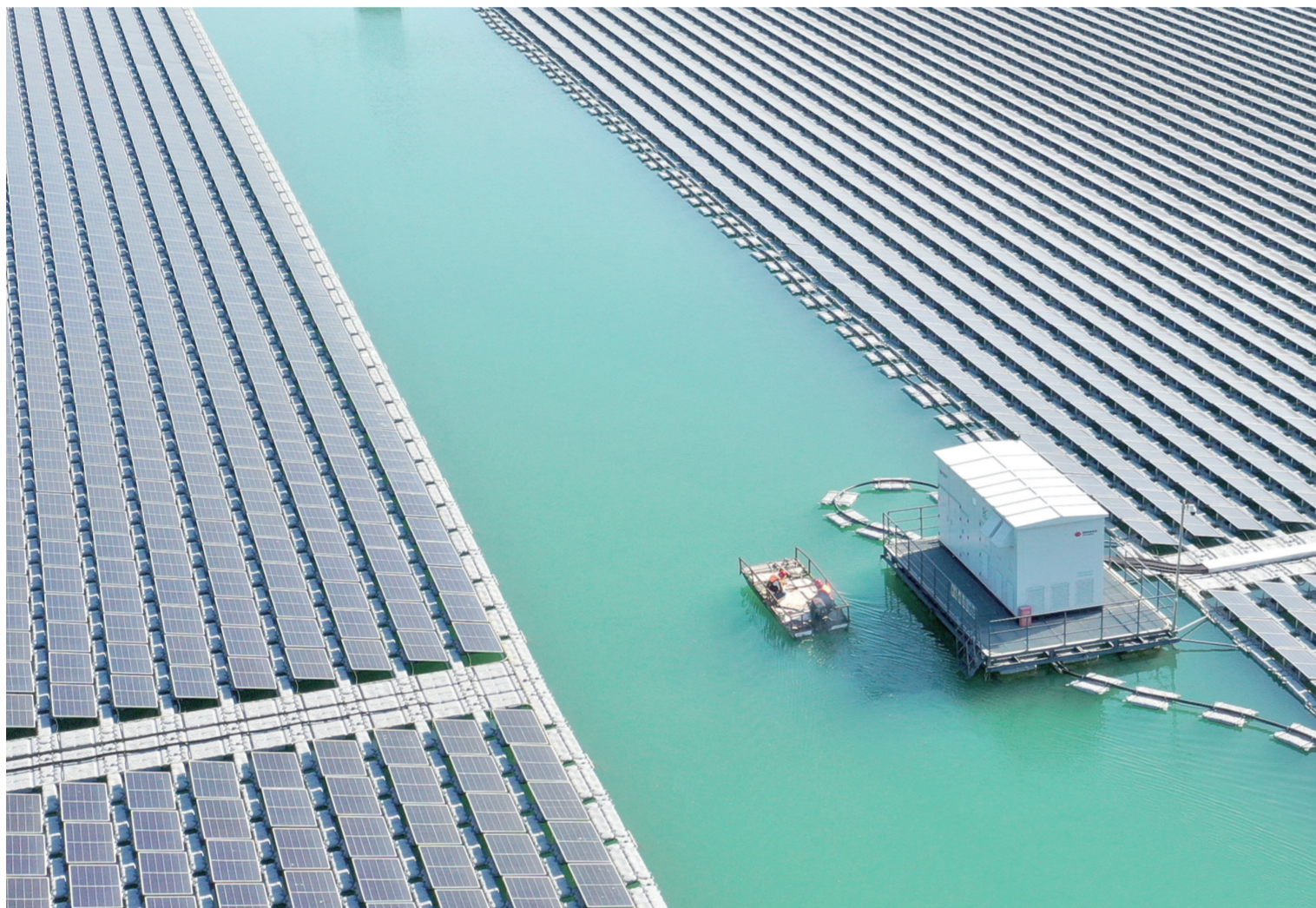
9月13日,在东昌府区堂邑镇固能聊城202兆瓦水库光伏项目现场,运维人员驾船对水上光伏进行巡检。该光伏电站投运以来,不断提高运维管理水平,全力以赴增发电量,经济效益、生态效益显著,为经济社会绿色低碳高质量发展注入新活力。 ■ 本报记者 许金松
